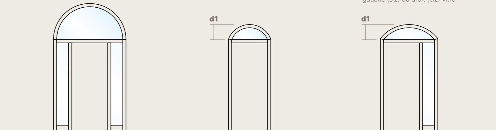
E2 Sopraluce con arco sesto ribassato e fiancoluce sinistro e destro Imposte cintrée vitrée et fixes latéraux vitrés
