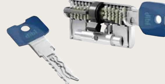
CILINDRO EUROPEO EVVA 3KS AD ALTISSIMA SICUREZZA CYLINDRE EUROPÉEN EVVA 3KS DE HAUTE SÉCURITÉ
