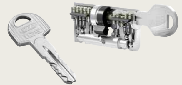
CILINDRO EUROPEO EVVA ICS AD ALTA SICUREZZA CYLINDRE EUROPÉEN EVVA ICS DE HAUTE SÉCURITÉ
