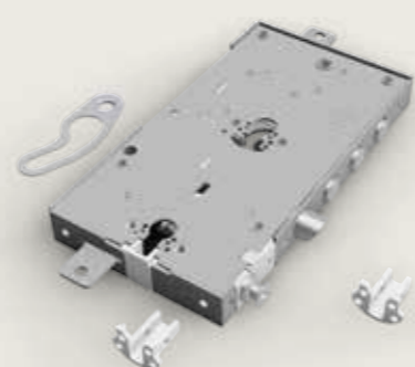
SERRATURA A INGRANAGGI SERRURE À ROUE DENTÉE
